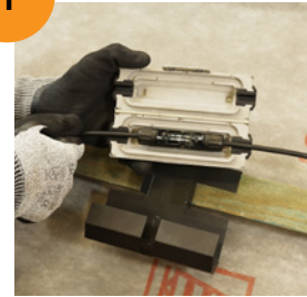
Plaats de MC4-connector in de behuizing met de kabels in de doorvoer
